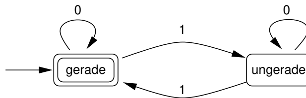
Abbildung 2: Ein endlicher Akzeptor zur Prüfung von Bitfolgen
