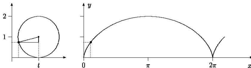
Abbildung 12.1.: Die Zykloide
