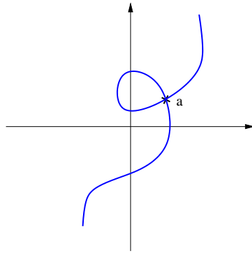
Abbildung 20.2.: Dies ist keine Untermannigfaltigkeit des \mathbb{R}^2 , denn diese Menge lässt sich in keiner Umgebung von a diffeomorph auf eine Strecke abbilden.
