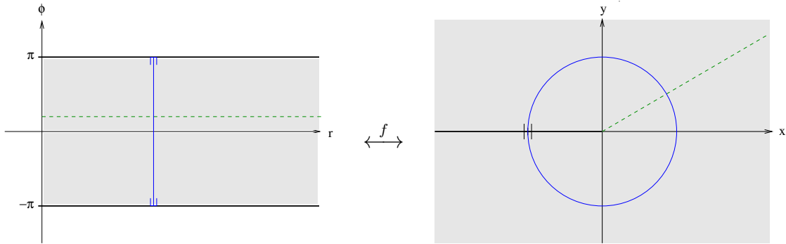
Abbildung 18.1.: Die Polarkoordinaten-Abbildung f bildet (0, \infty) \times (-\pi, \pi) diffeomorph auf \mathbb{R}^2 \setminus \{(x, 0) : x \leq 0\} ab, ist aber auf (0, \infty) \times \mathbb{R} nicht bijektiv.
