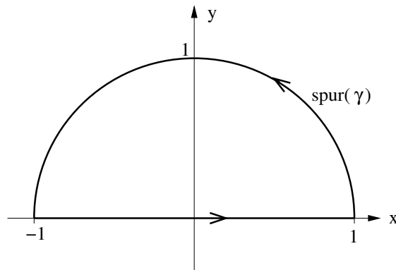
Abbildung 23.1.: Der Weg \gamma aus Beispiel 23.10
