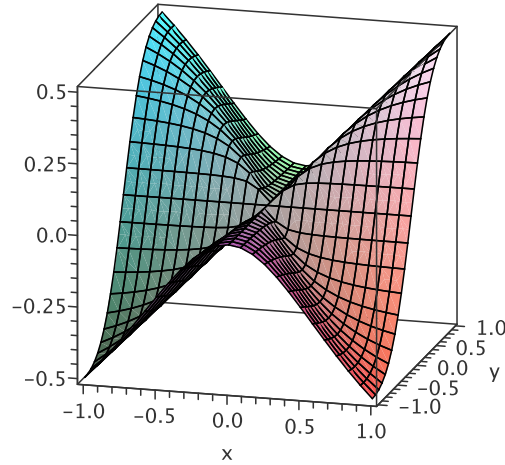
Abbildung 8.2.: Der Graph der Funktion (x, y) \mapsto \frac{x^2 y}{x^2 + y^2}
