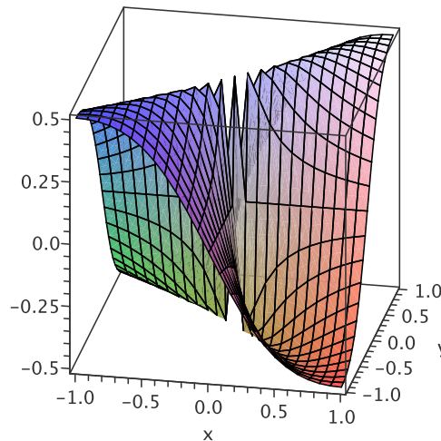
Abbildung 8.1.: Der Graph der Funktion (x, y) \mapsto \frac{xy}{x^2+y^2}
