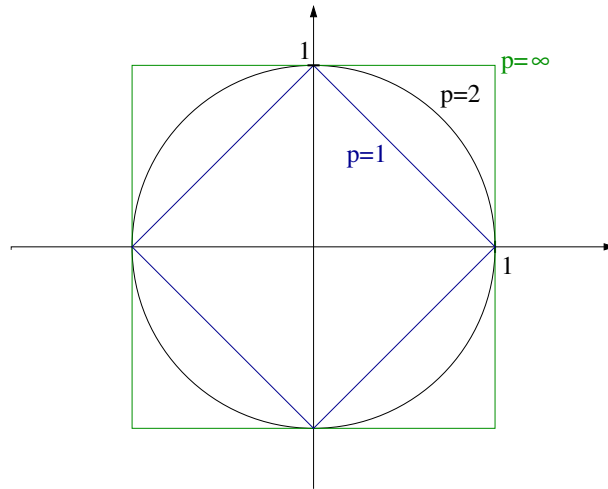
Abbildung 4.1.: Die Ränder der Einheitskugeln im \mathbb{R}^2 für die 1-, 2- und \infty -Norm
