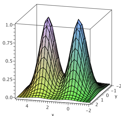
Abbildung 17.2.: Der Graph der Funktion f(x, y) = e^{-x^2-y^2} + e^{-(x-3)^2-y^2}
