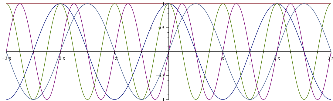
Abbildung 1.1.: Die ersten fünf Fourier-Basis-Funktionen 1 , \cos(x) , \cos(2x) , \sin(x) und \sin(2x) .
