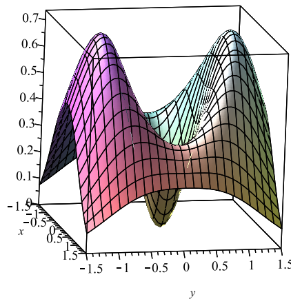
Abbildung 17.1.: Der Graph der Funktion f(x, y) = (x^2 + 2y^2)e^{-x^2 - y^2}
