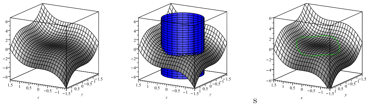
Abbildung 21.1.: Links der Graph der Funktion f(x, y) = x^3 - y^3 , in der Mitte der selbe Graph mit dem Zylinder, dessen Rand genau S^1 ist. Rechts die Schnittlinie des Zylinders mit dem Graphen. Der Maximalwert von f auf S^1 entspricht dem höchsten Punkt auf dieser grünen Linie.
