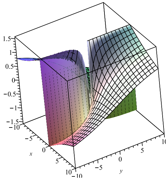
Abbildung 23.2.: Der Graph der Funktion \varphi(x, y) = \arctan(y/x) ist entlang der gesamten y -Achse unstetig.
