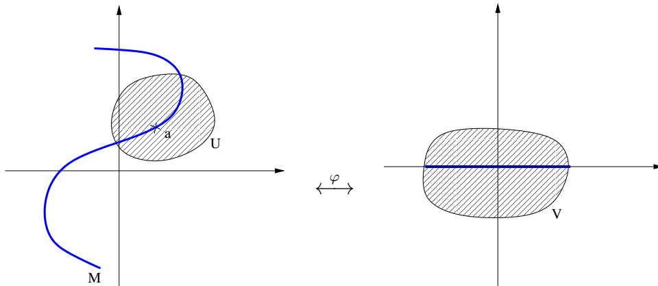
Abbildung 20.1.: Definition einer Untermannigfaltigkeit: In einer Umgebung von a lässt sich die eindimensionale Untermannigfaltigkeit M des \mathbb{R}^2 zu einem geraden Stück \mathbb{R} diffeomorph glattziehen.
