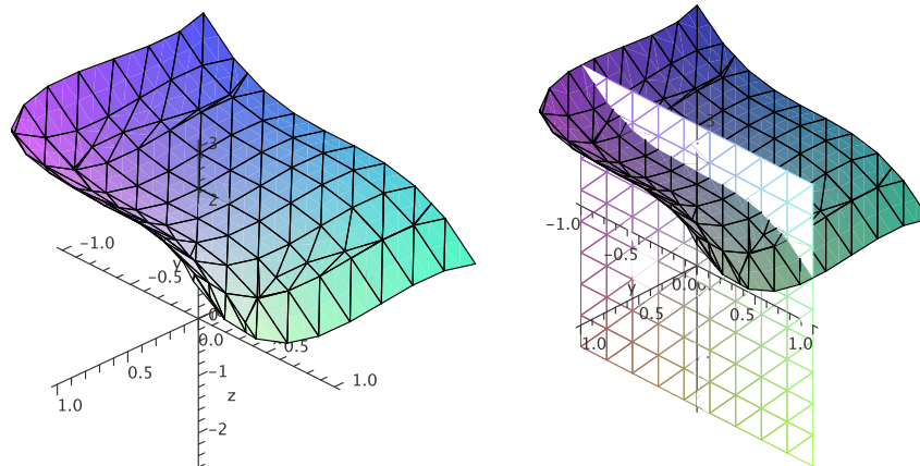
Abbildung 13.1.: Der Graph einer Funktion von \mathbb{R}^2 nach \mathbb{R} und der Schnitt, der zu einer partiellen Ableitung, d. h. Richtungsableitung in Richtung einer Koordinatenachse, führt
