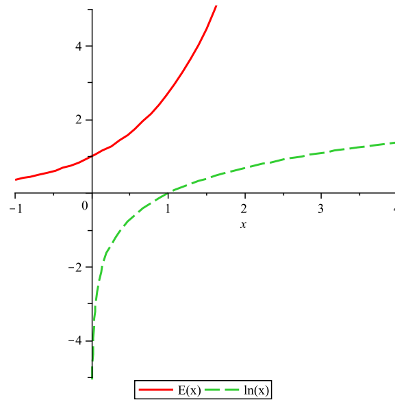
Abbildung 19.2.: Die Graphen der Exponentialfunktion und des Logarithmus
