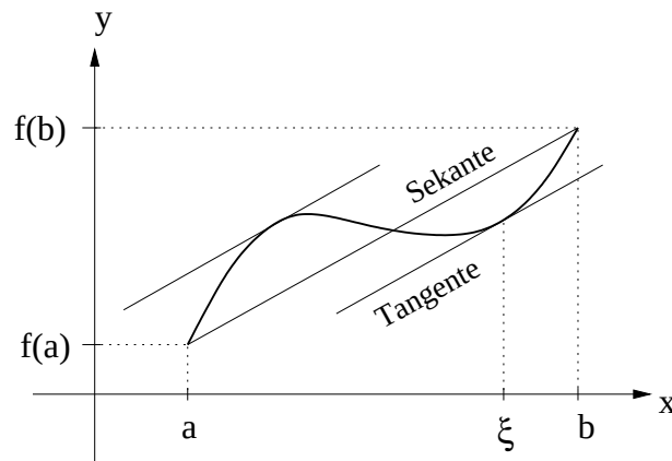
Abbildung 22.1.: Der Mittelwertsatz der Differenzialrechnung
