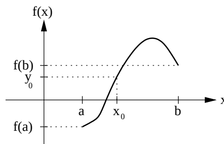
Abbildung 19.1.: Der Zwischenwertsatz
