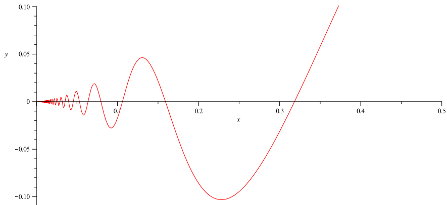
Abbildung 24.1.: Der Graph des „Flattersinus“ aus Beispiel 24.2 (d)
