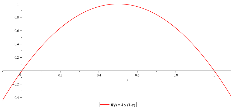
Abbildung 3.1: Die Funktion f(y) = \mu y(1 - y) mit \mu = 4 .
