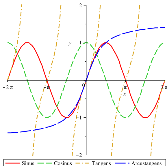
Abbildung 26.2.: Die Graphen von Sinus, Cosinus, Tangens und Arcustangens
