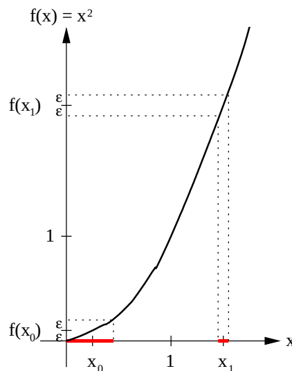
Abbildung 22.1.: Die Abhängigkeit des Stetigkeits-Deltas von x_0
