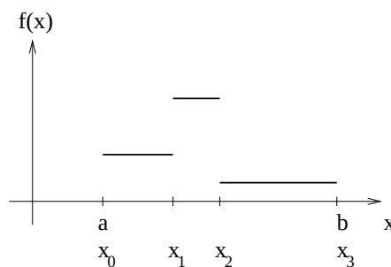
Abbildung 29.2.: Beispiel einer Treppenfunktion
