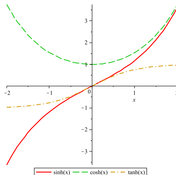
Abbildung 26.3.: Die Graphen von Sinus, Cosinus und Tangens hyperbolicus
