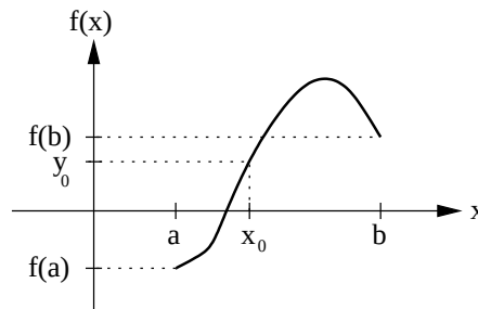
Abbildung 20.1.: Der Zwischenwertsatz
