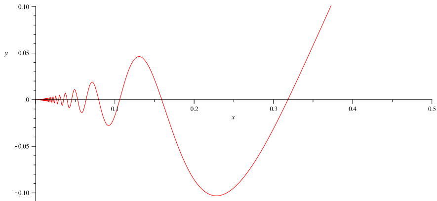
Abbildung 27.1.: Der Graph des „Flattersinus“ aus Beispiel 27.2 (d)
