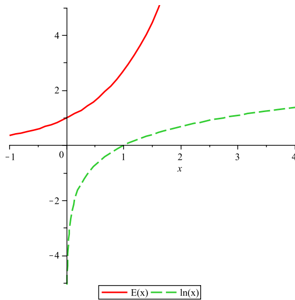
Abbildung 20.2.: Die Graphen der Exponentialfunktion und des Logarithmus
