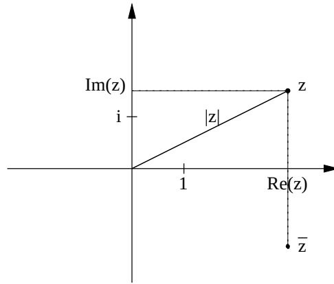
Abbildung 17.1.: Die Gaußsche Zahlenebene
