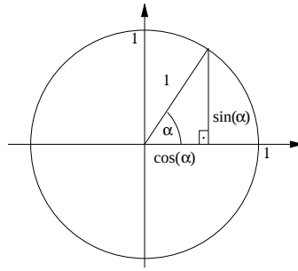
Abbildung 26.1.: Trigonometrischer Pythagoras
