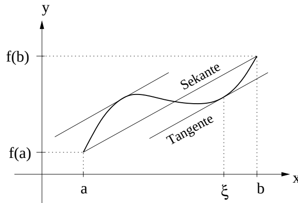
Abbildungung 24.1.: Der Mittelwertsatz der Differenzialrechnung
