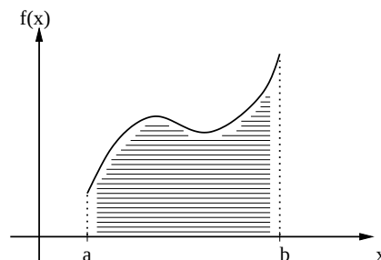
Abbildung 29.1.: Zu bestimmende Fläche unter dem Funktionsgraphen
