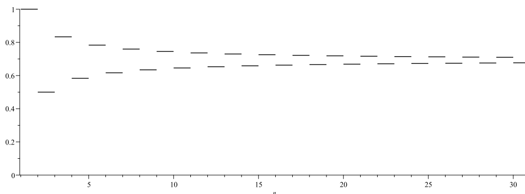
Abbildung 12.1.: Die ersten dreißig Partialsummen der alternierenden harmonischen Reihe.
