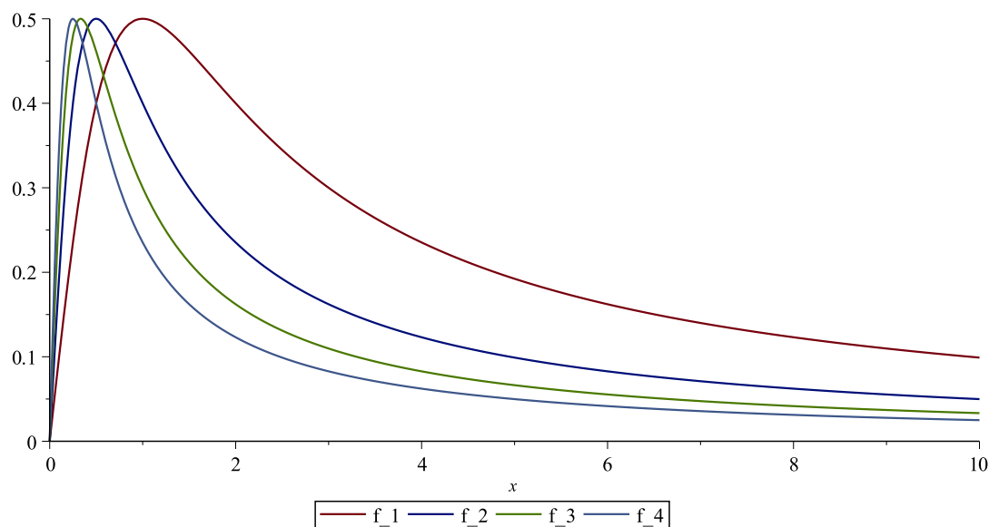
Abbildung 21.1.: Die Graphen der ersten vier Funktionen in der Funktionenfolge aus Beispiel 21.2 (c).
