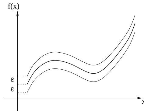
Abbildung 21.2.: Der \varepsilon -Streifen um den Graphen der Grenzfunktion f .
