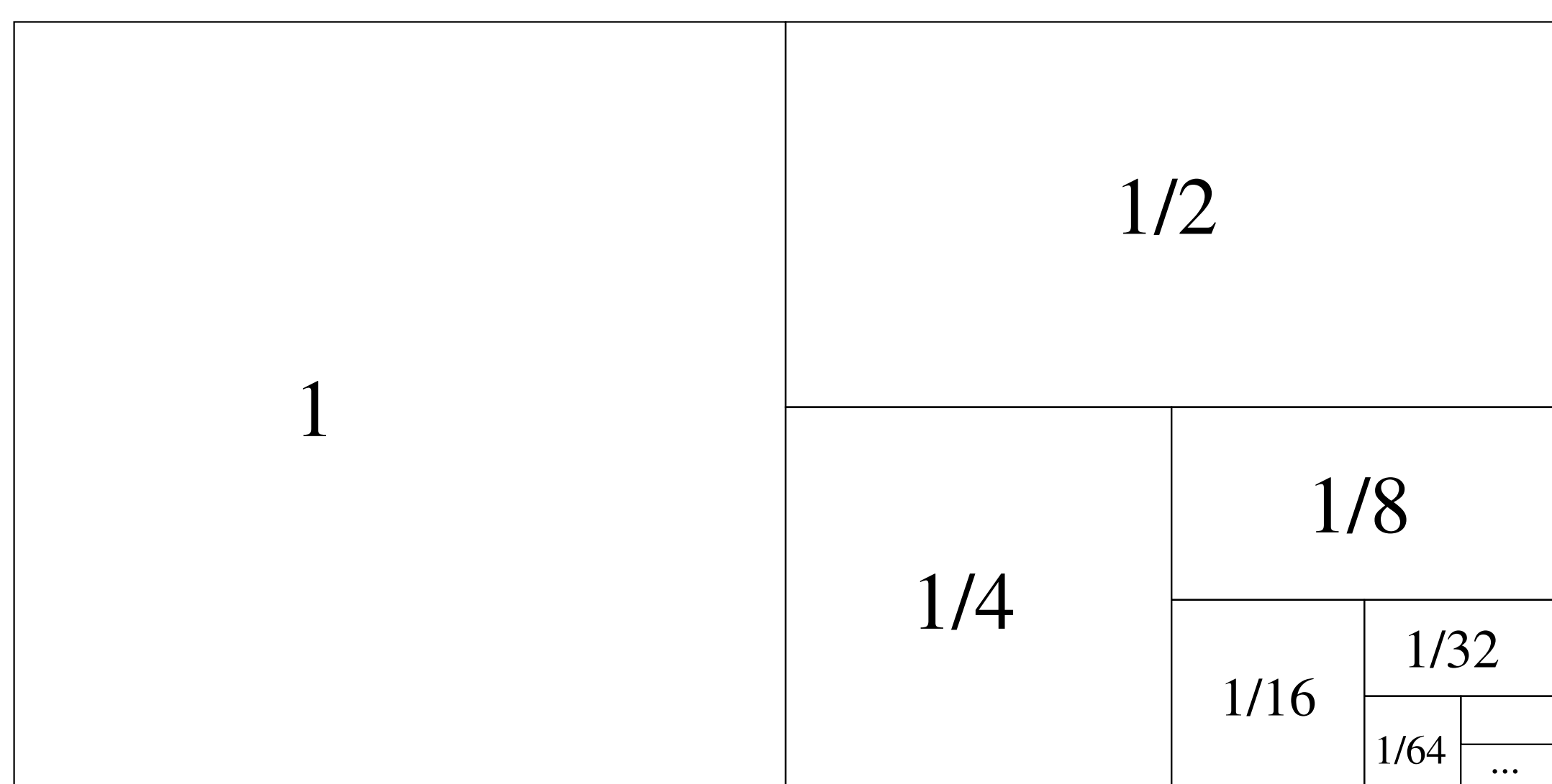
Abb. 1: Veranschaulichung der geometrischen Reihe
