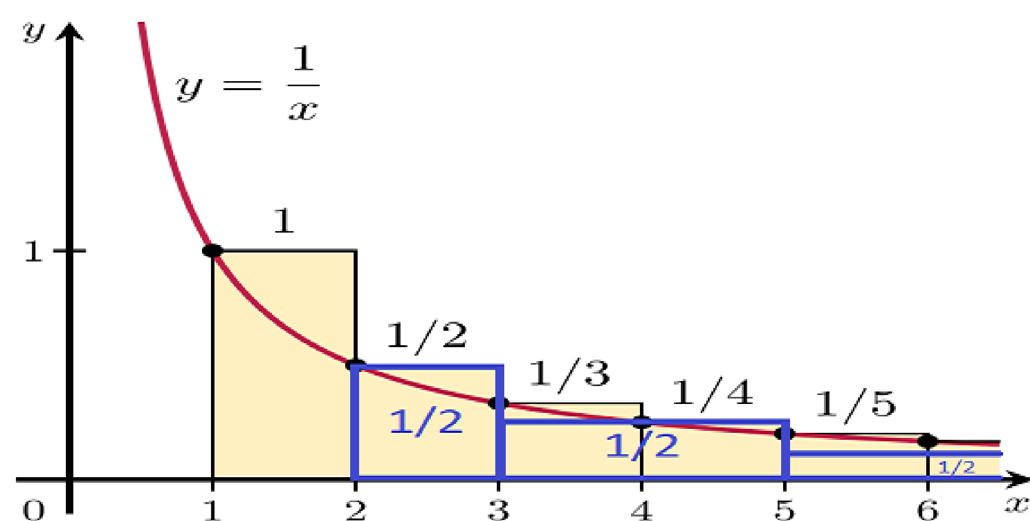
Abb. 2: Illustration der harmonischen Reihe
